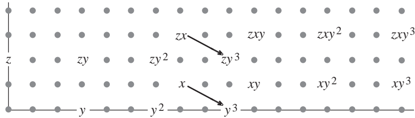
The E_2 -term
